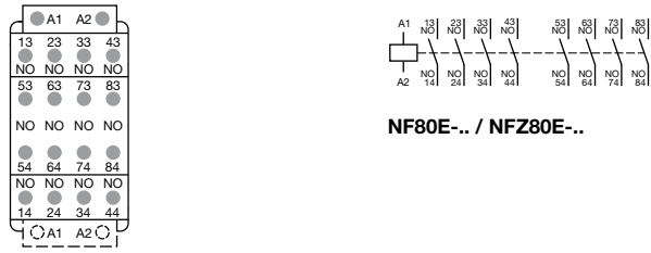
NF80E-.. / NFZ80E-..
